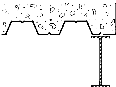
POUR STOP AT SIDE
