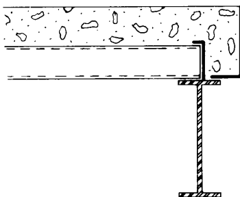
POUR STOP AT END
